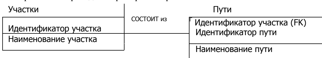
Рис. 11. Идентифицирующая связь
