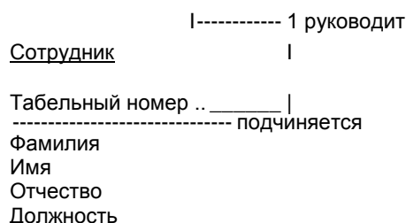
Рис. 13. Рекурсивная связь
