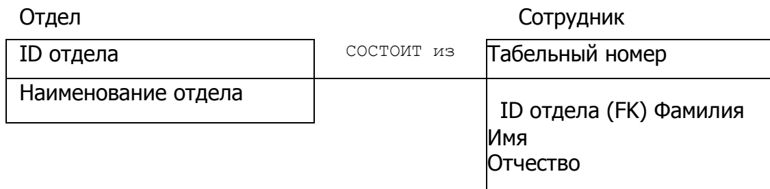
Рис. 12. Неидентифицирующая связь
