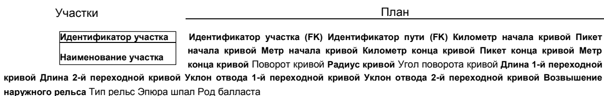
Рис. 10. Сущности
