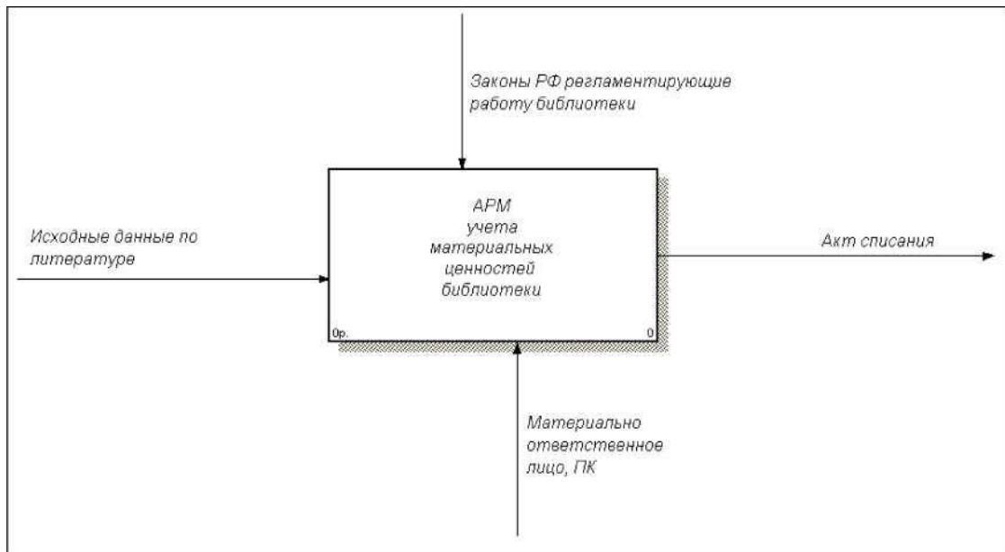
Рис.1. Контекстная диаграмма
