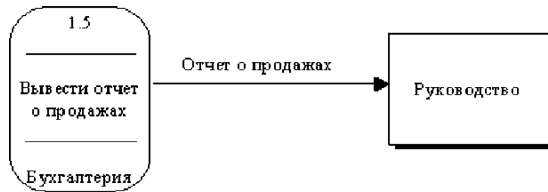
Рис. 7. Поток данных
