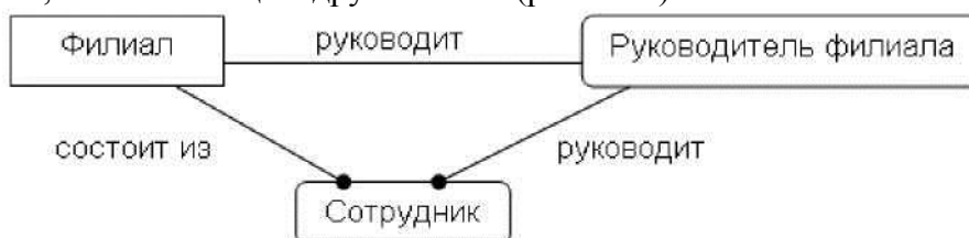
Рис. 18. Избыточные связи
