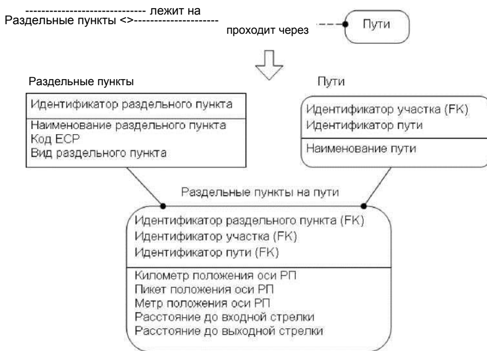
Рис. 15. Замена связи N:M
